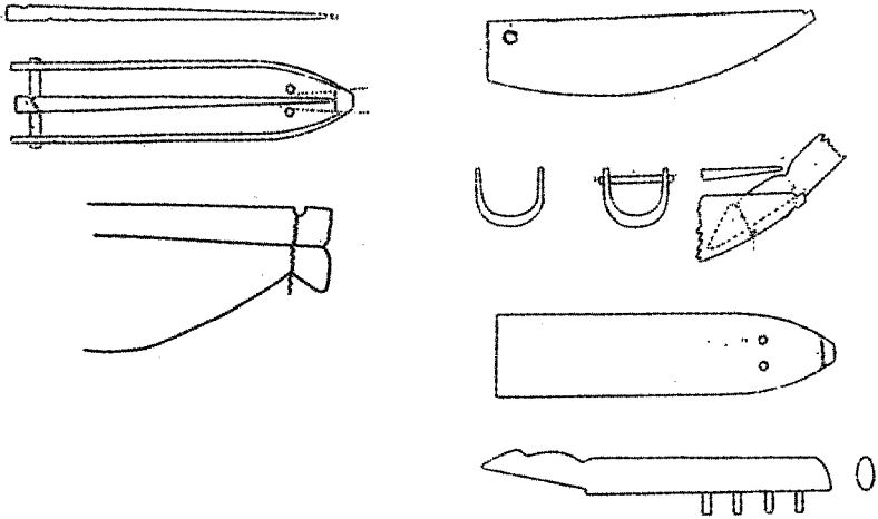
(شكل : ٢٨٧) تركيب صندوق صوتي لهارب ورقبته، دولة حديثة
